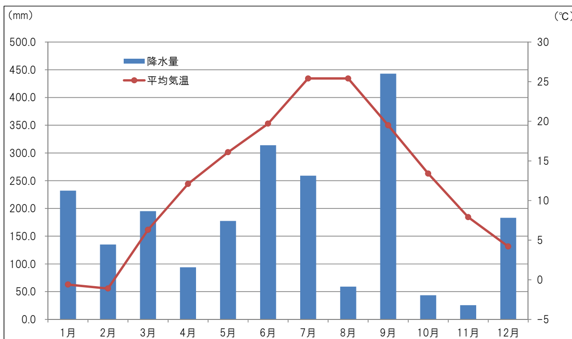
図 1-4 月別降水量・月別平均気温（平成 30 年）
