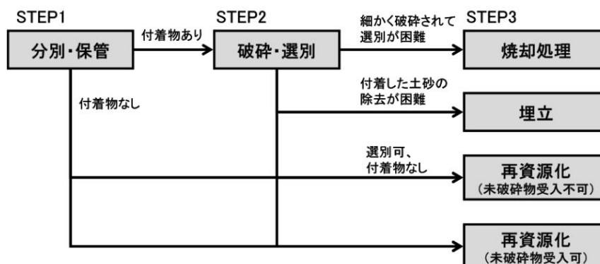
図 2-12 木質系廃棄物の処理フロー
